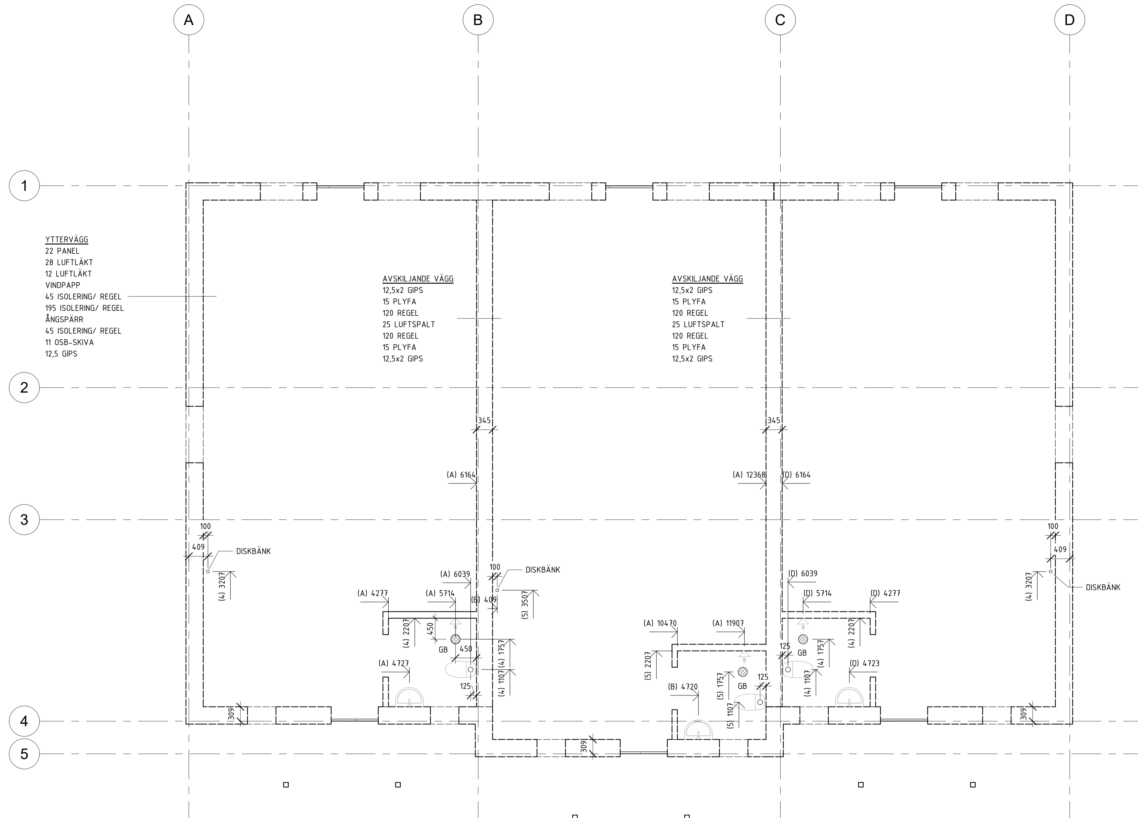
AVSÄTTNINGSPLAN 1 : 50
