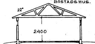
SEKTION
