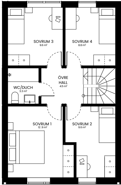
ÖVRE PLAN
