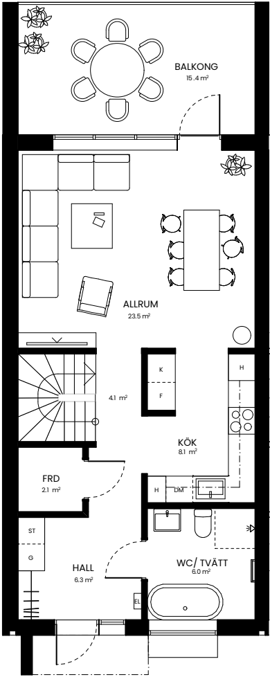
ENTRÉPLAN
