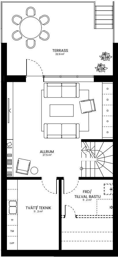
SUTERRÄNGPLAN
