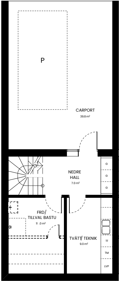
SUTERRÄNGPLAN
