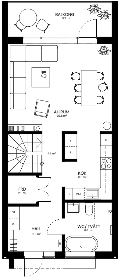
ENTRÉPLAN
