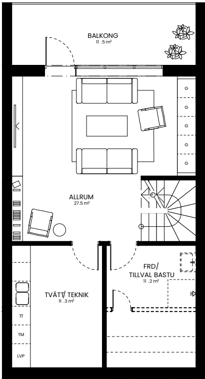
SUTERRÄNGPLAN
