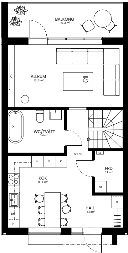
ENTRÉPLAN
