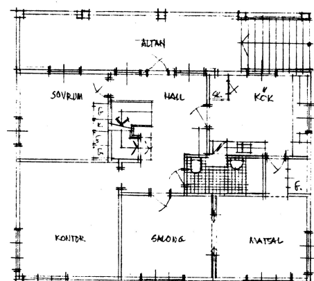
BOTTENVÅNING
