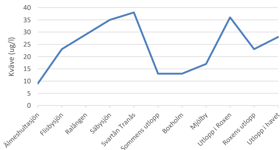
Figur 6. Sommen och de strömmande vattnen svarar för en rening av vattnet från närsalterna fosfor och kväve. När de förekommer i överskott är vattnet övergött (eutrofierat) och flora och fauna förändras. I figuren ser vi hur vatten i Svartån förändras från källorna (till vänster) ned till mynningen i havet (till höger). Halterna av fosfor ökar i jordbrukslandskapet och får ett tillskott från reningsverk på sträckan Aneby ned till Tranås. Men när vattnet kommer ut från Sommen har det förändrats radikalt, en reningsprocess som förbättrar vattenkvaliteten långt nedströms. Bidragande i lika stor utsträckning är också ett tillskott av vatten av bättre vattenkvalitet från Bulsjön genom västra Sommen. Modellerade närsalthalter från SMHI Vattenweb för åren 2010–2019.
