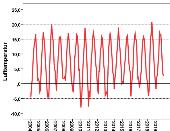
Figur 11. Lufttemperatur vid Sömmens utlopp, Laxberg, angivet som månadsmedelvärden 2004–2019 enligt SMHI.
