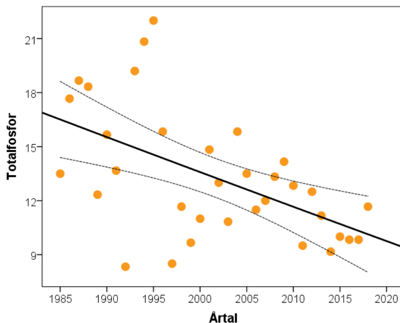
Figur 13. Uppmätta halter (mikrogram per liter; \mu\text{g/l} ) av totalfosfor under april-oktober i ytvatten (0,5–3 m) 1985–2019 i Sommens utlopp. Kraftigare linje markerar linjär trend och streckade linjer dess osäkerhetsintervall (95%-konfidensintervall). Data Motala Ströms Vattenvårdsförbund.
