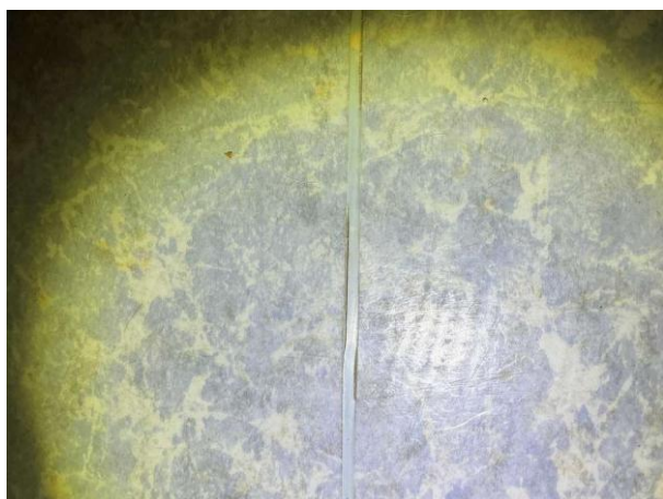
Bild 3: - Invändigt, Soutterrängplan, Äldre våtrum med plastmatta på golvet Sprickor noteras vid matskarven Det förekommer Rör genomföring...
