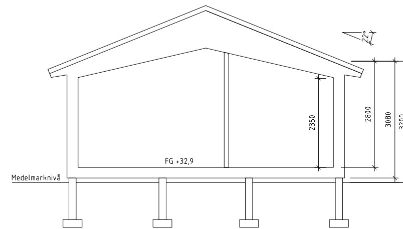
Sektion A-A
