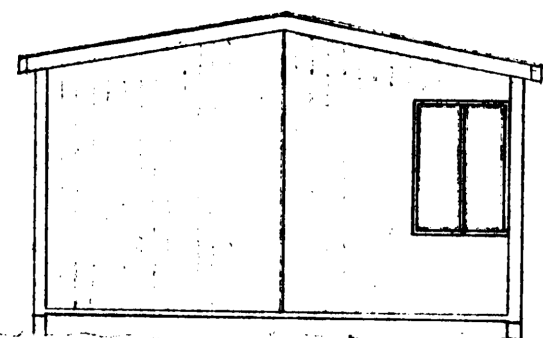
FASAD 1. 1:50
