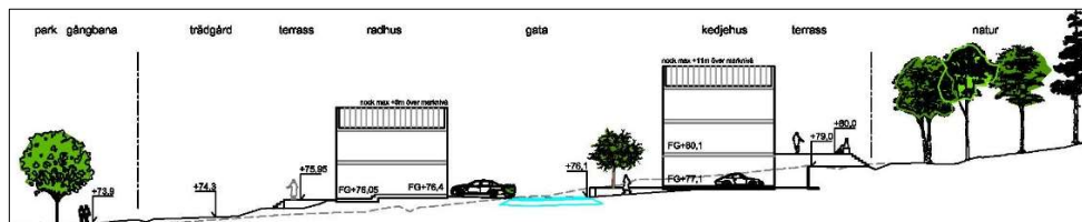
Anpassning till områdets topografiska förhållanden med kuperad terräng. Nybebyggelse placeras mellan parkstråk i väst och bergssluttning i öst. Illustration Studio M2L
